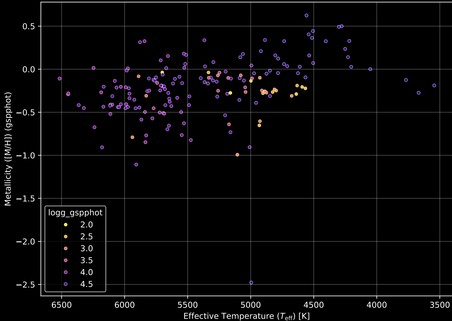
APOGEE DR17 Field: [JHelum3] Stellar Population Parameters (n= 175)
